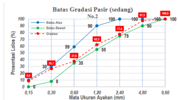
Gambar 2 Grafik uji gradasi agregat halus
